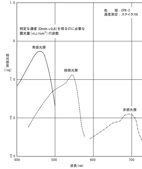
分光感度曲線
